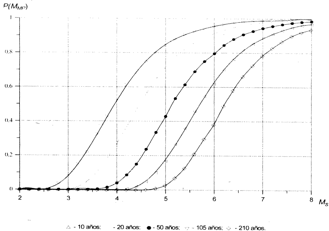
Figura 4. Probabilidad de no-excedencia de magnitud máxima probable M_{mp} para los tiempos de exposición
