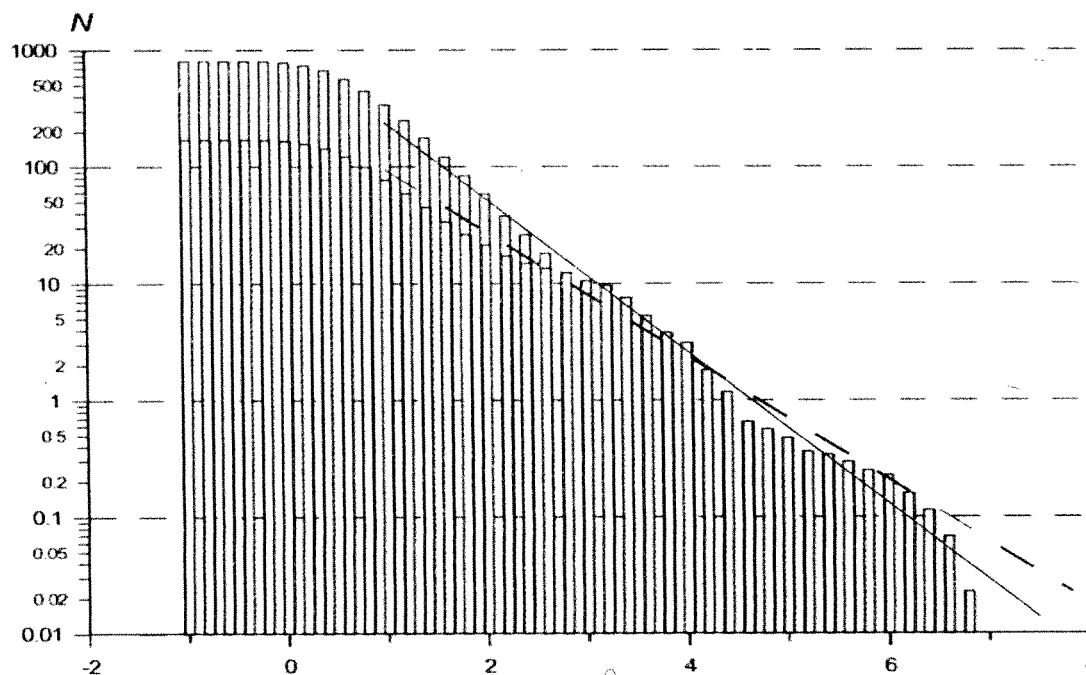
Figura 2. Gráfico de recurrencia acumulativa para la región en estudio, para el intervalo de tiempo 1958-2002
