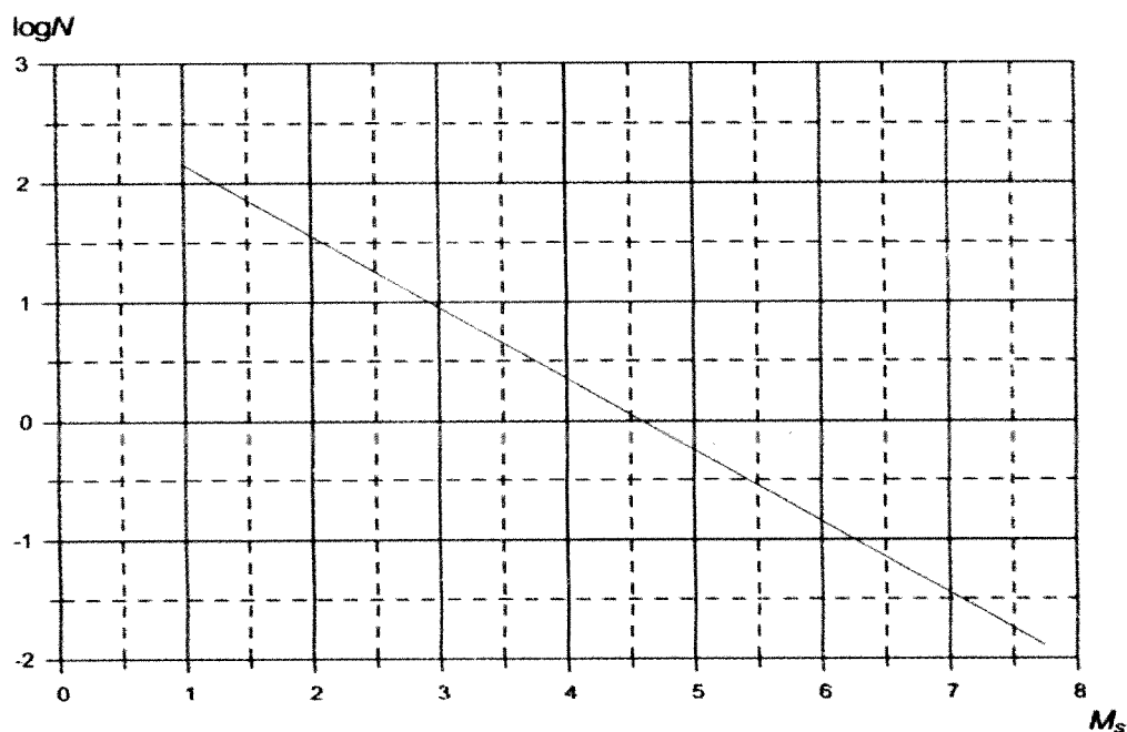
Figura 3. Regresión correspondiente al gráfico de recurrencia de la base de datos artificial. \log N = -0.601M + 2.76
