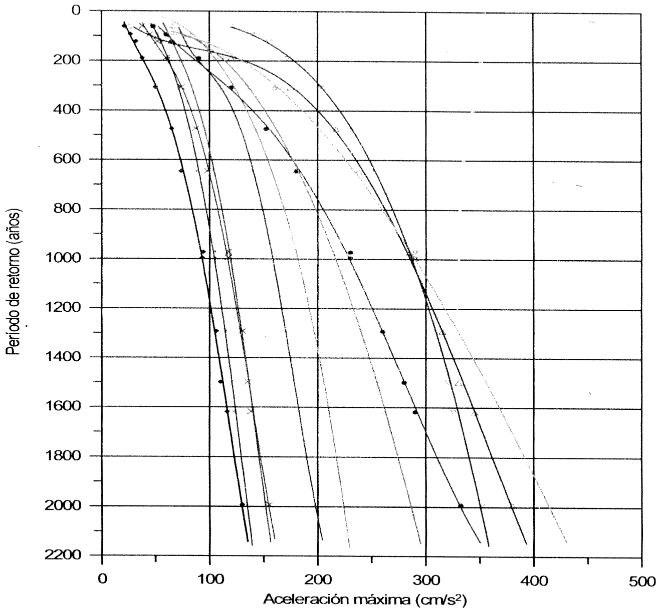
Figura 6. Aceleración máxima probable a_{max} para diversos valores del período de retorno promedio T_R
