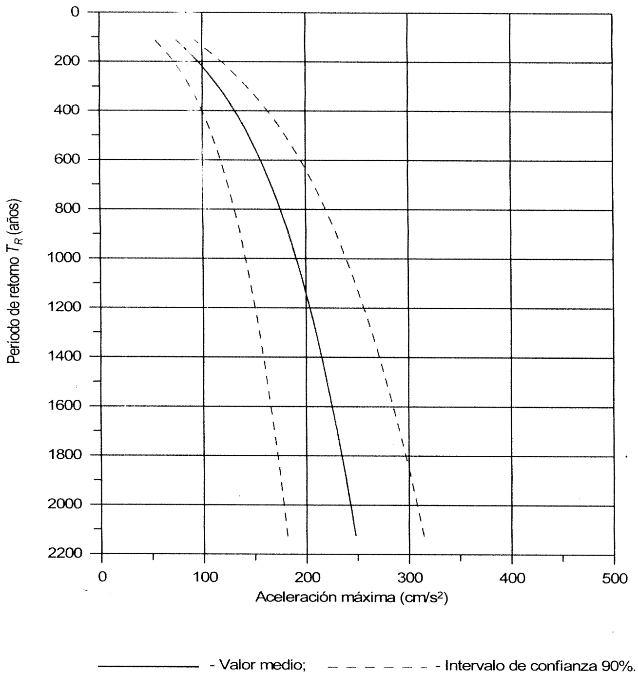
Figura 7. Aceleración máxima probable a_{m\acute{a}x} (valor medio) para diversos valores de periodo de retorno promedio T_R
