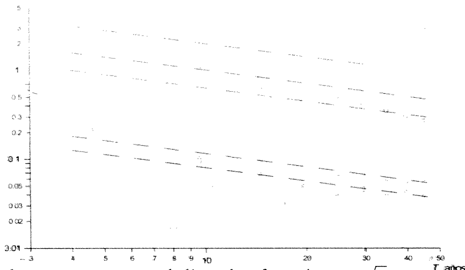
Figura 1. Completitud. Desviación estándar \sigma del número anual medio de eventos en función de la extensión de la muestra.
