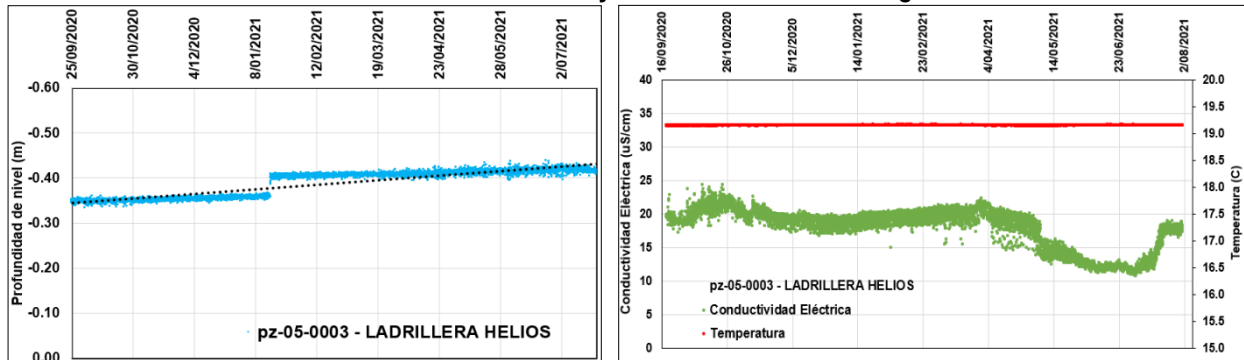
Figura 12. Comportamiento del nivel estático, temperatura y conductividad eléctrica del pozo pz-05-0003- Acuitardo Formación Usme y Acuitardo Formación Regadera.
