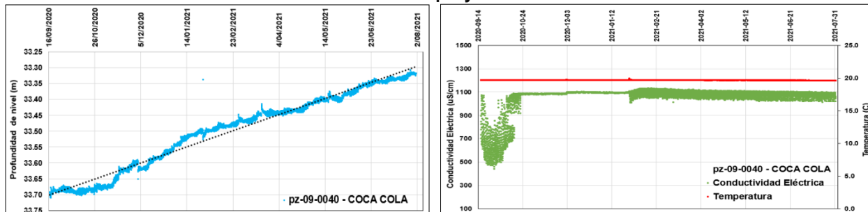
Figura 19. Comportamiento del nivel estático, temperatura y conductividad eléctrica del pozo pz-09-0040- Acuitarfo Formación Subchoque y Acuífero Formación Tilatá.
