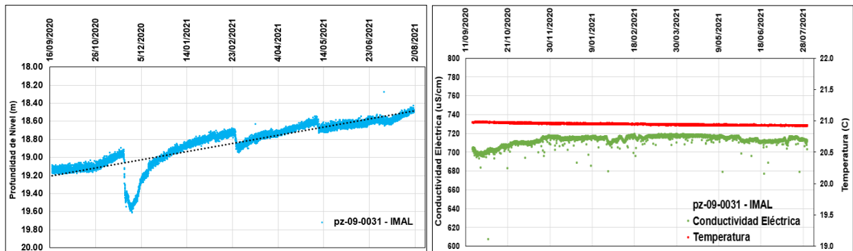
Figura 17. Comportamiento del nivel estático, temperatura y conductividad eléctrica del pozo pz-09-0031- Acuífero Formación Sabana-Tilatá.
