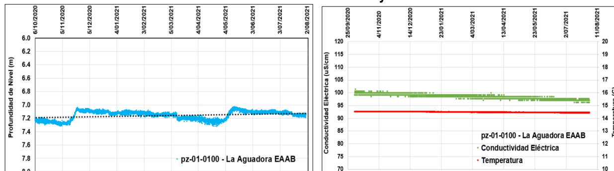
Figura 11. Comportamiento del nivel estático, temperatura y conductividad eléctrica del pozo pz-01-0100- Acuífero Formación Labor-Tierna y Plaeners.
