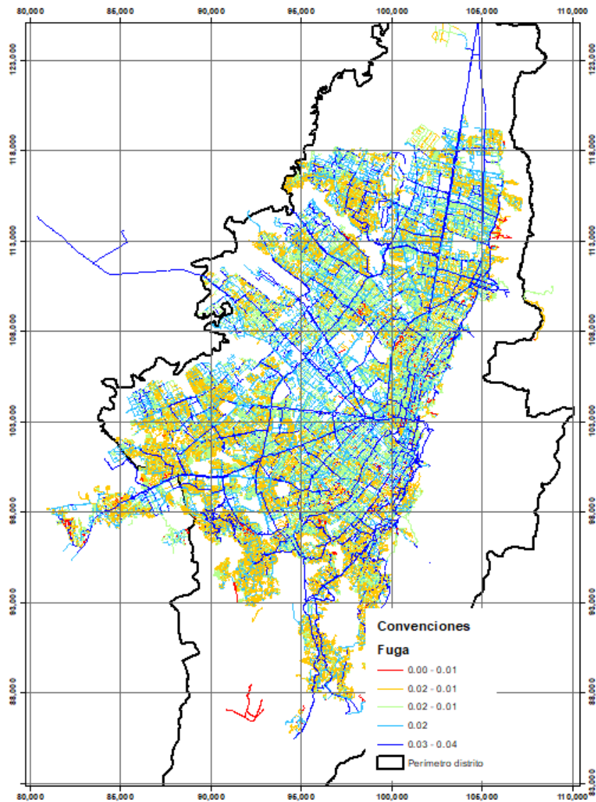
Figura 4-38: Fugas en l/s red de acueducto
