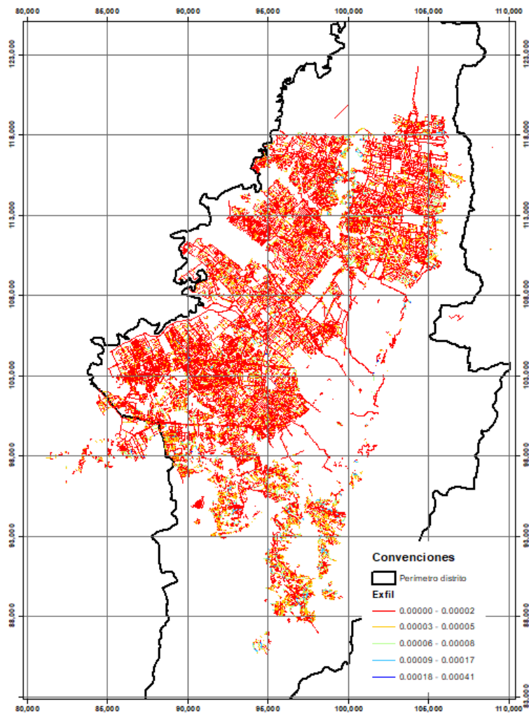
Figura 4-40: Exfiltraciones en m 3 /s de la red de alcantarillado pluvial
