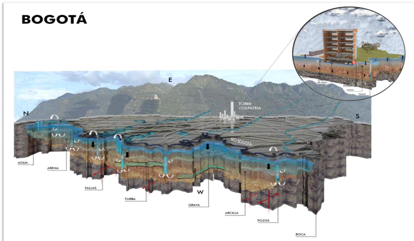
Figura 5-22 Representación gráfica del modelo hidrogeológico conceptual.
