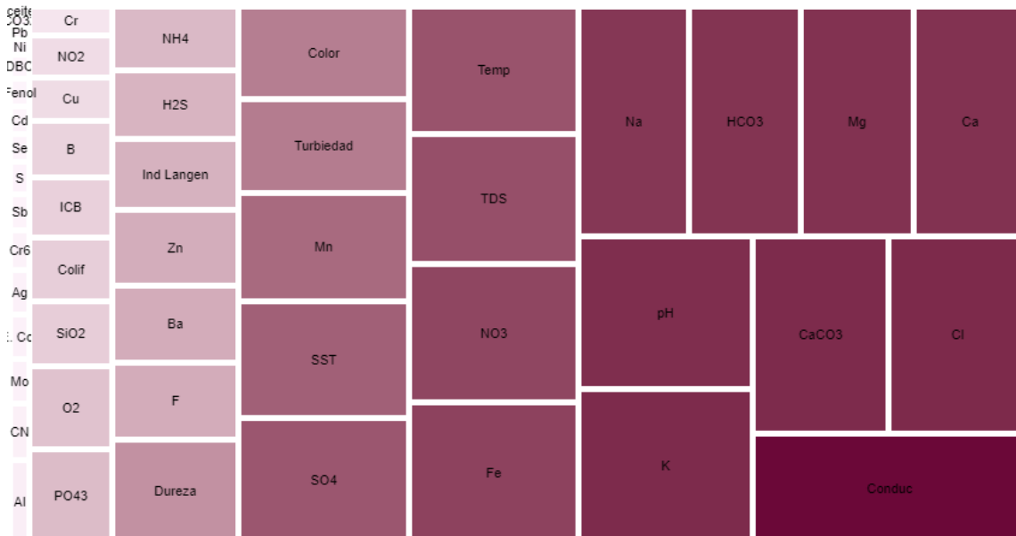
Figura 4-8 Proporción de parámetros hidroquímicos en el depósito no consolidado
