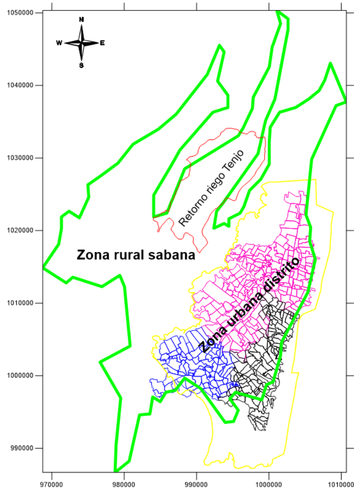
Figura 5-10 Áreas de recarga consideradas para el balance hídrico global.
