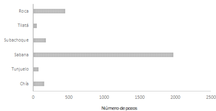
Figura 3-21 Número de pozos que atraviesan las formaciones geológicas de los depósitos cuaternarios y del basamento rocoso
