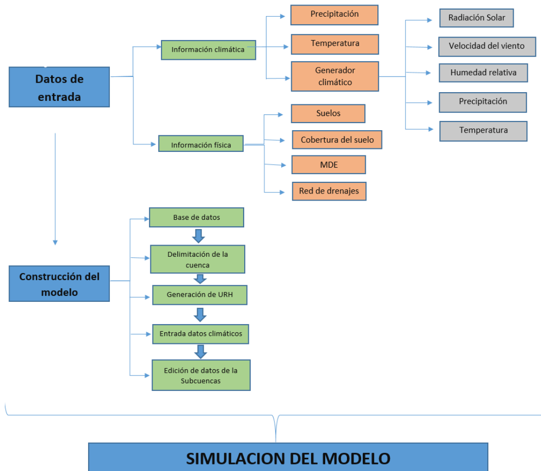
Figura 4-36 Metodología de la aplicación del modelo
