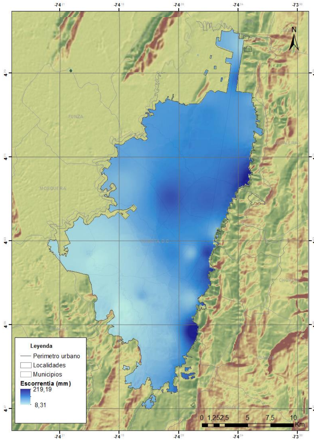
Figura 3-10 Mapa de Escorrentía superficial
