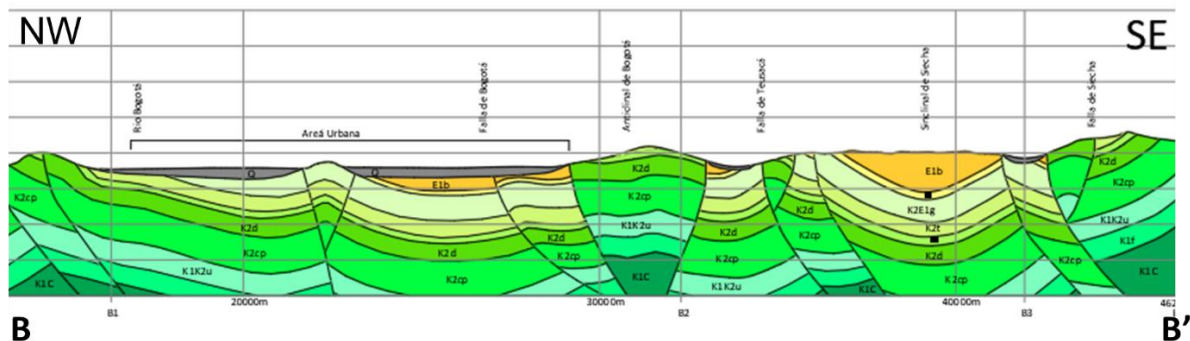
Figura 4-11. Perfil Geológico corte B-B'
