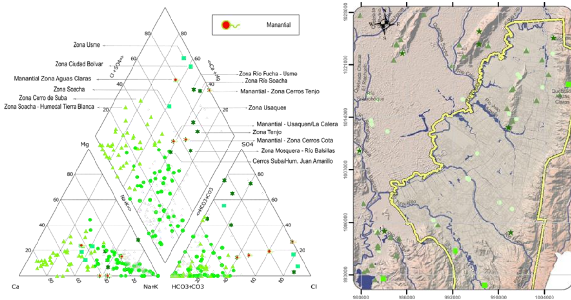
Figura 3-25 Tipos de agua encontrados en los puntos de agua que atraviesan el basamento rocoso
