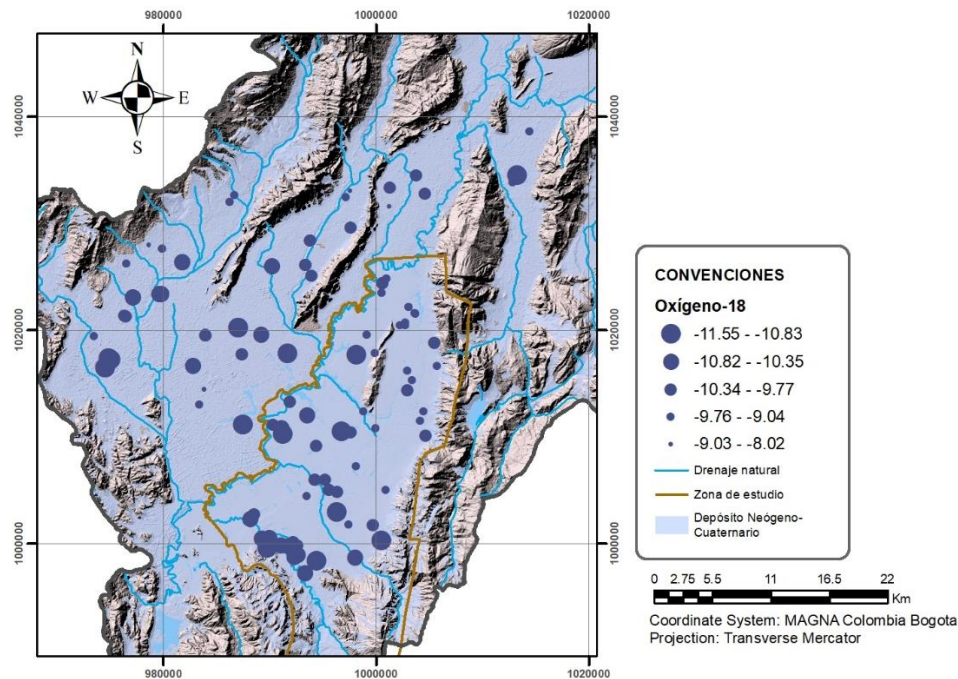
Figura 4-7 Puntos de agua con información de oxígeno-18 – Depósito no consolidado
