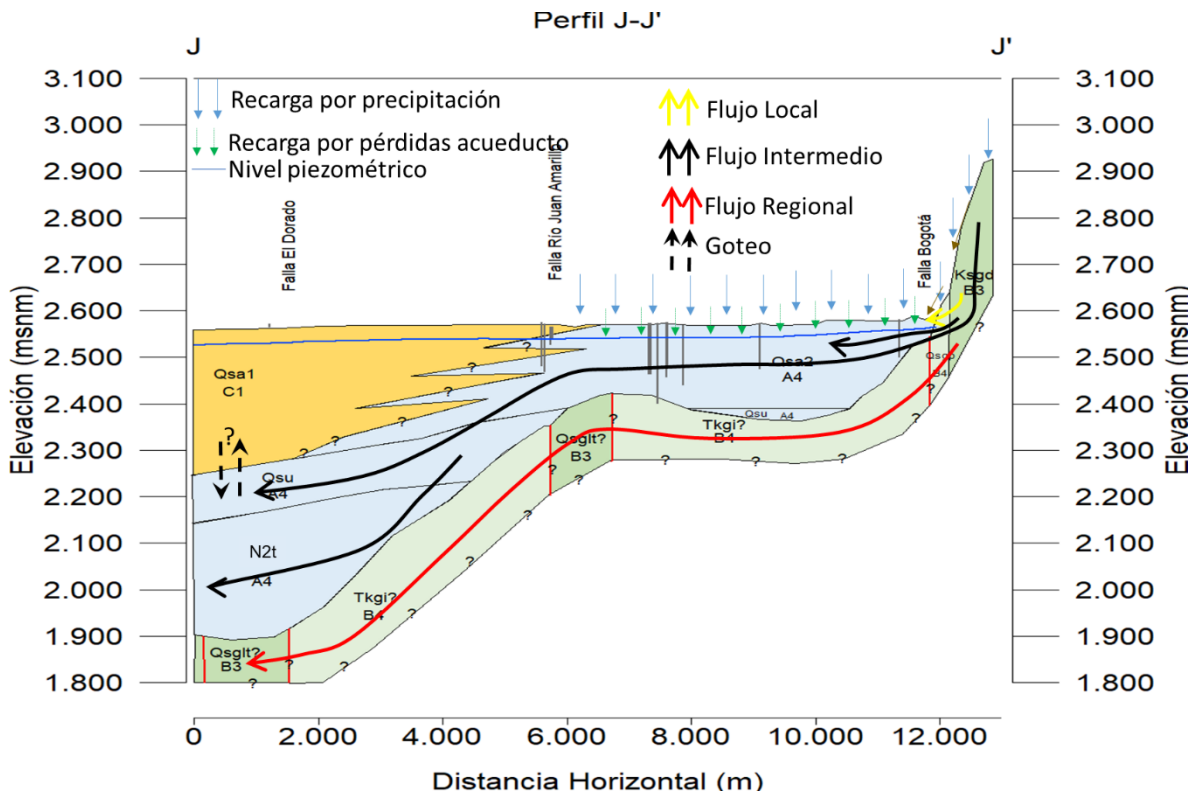
Figura 5-20. Representación gráfica del perfil hidrogeológico J-J'
