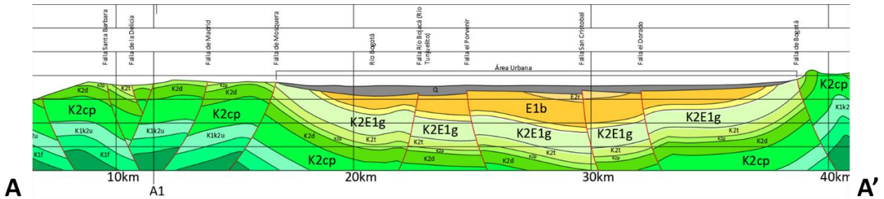
Figura 4-9. Perfil Geológico corte A-A'
