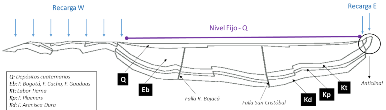
Figura 4-10. Dominio y representación del modelo analítico de flujo 2D, perfil geológico A-A'
