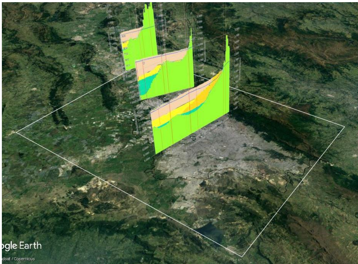
Figura 4-35 Perfiles estratigráficos G-G', J-J', O-O'; exagerados 10 veces en la vertical superpuesto sobre imagen de Google earth.
