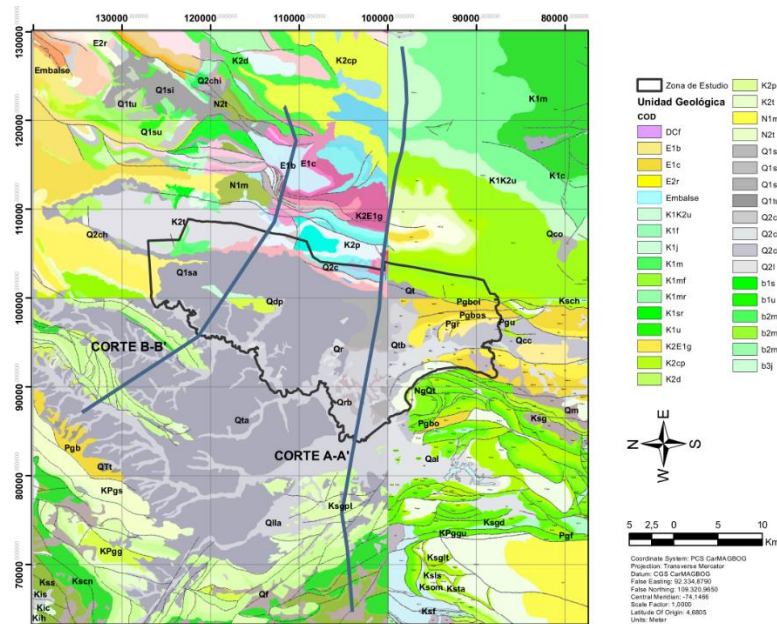
Figura 4-42. Dominio del modelo analítico de flujo 2D, perfil geológico A-A'
