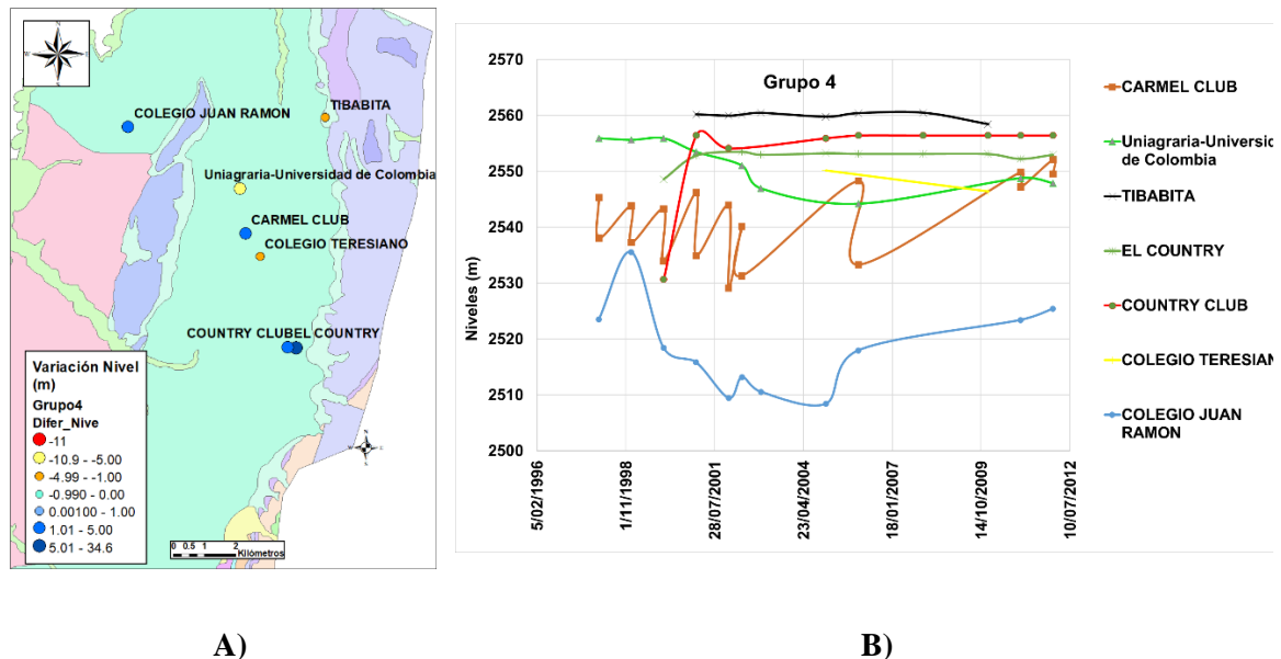
Figura 5-8. Localización y evolución temporal de los pozos localizados en el grupo 4. A). Localización y el valor puntual entre la diferencia de nivel medido entre la más reciente a la más antigua, B). Evolución temporal de los niveles.
