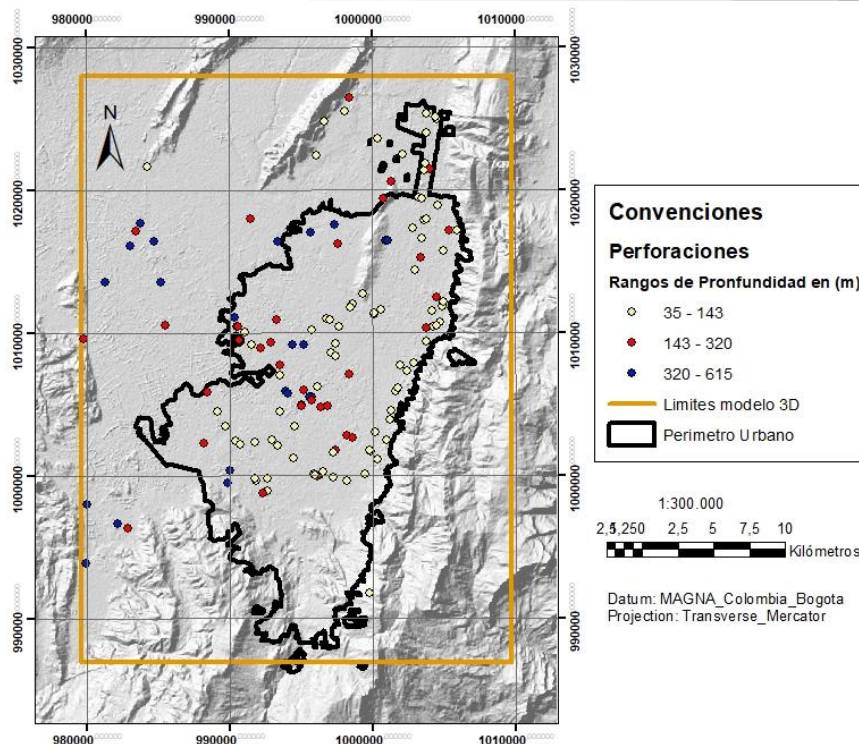
Figura 4-25. Distribución en superficie de las perforaciones usadas para la construcción del modelo 3D
