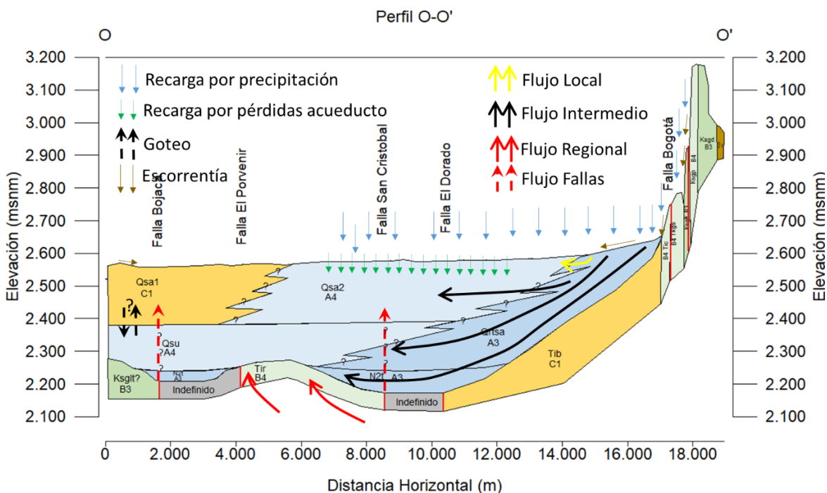
Figura 5-19 Representación gráfica del perfil hidrogeológico O-O'
