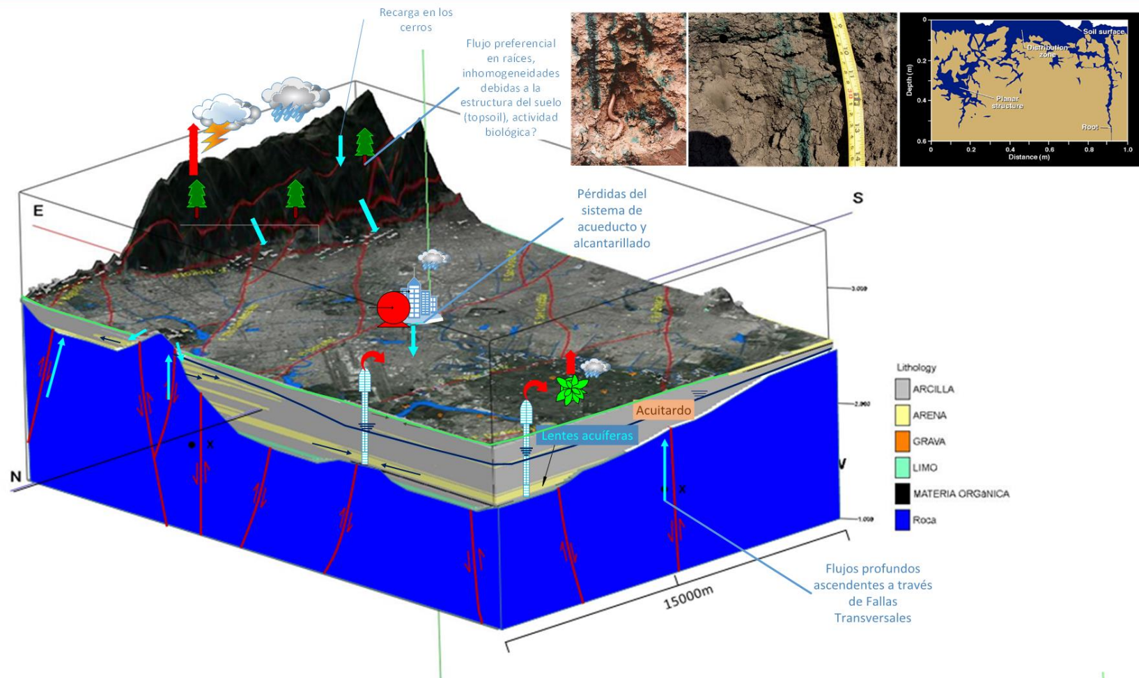
Figura 5-21. Representación gráfica del modelo hidrogeológico conceptual.
