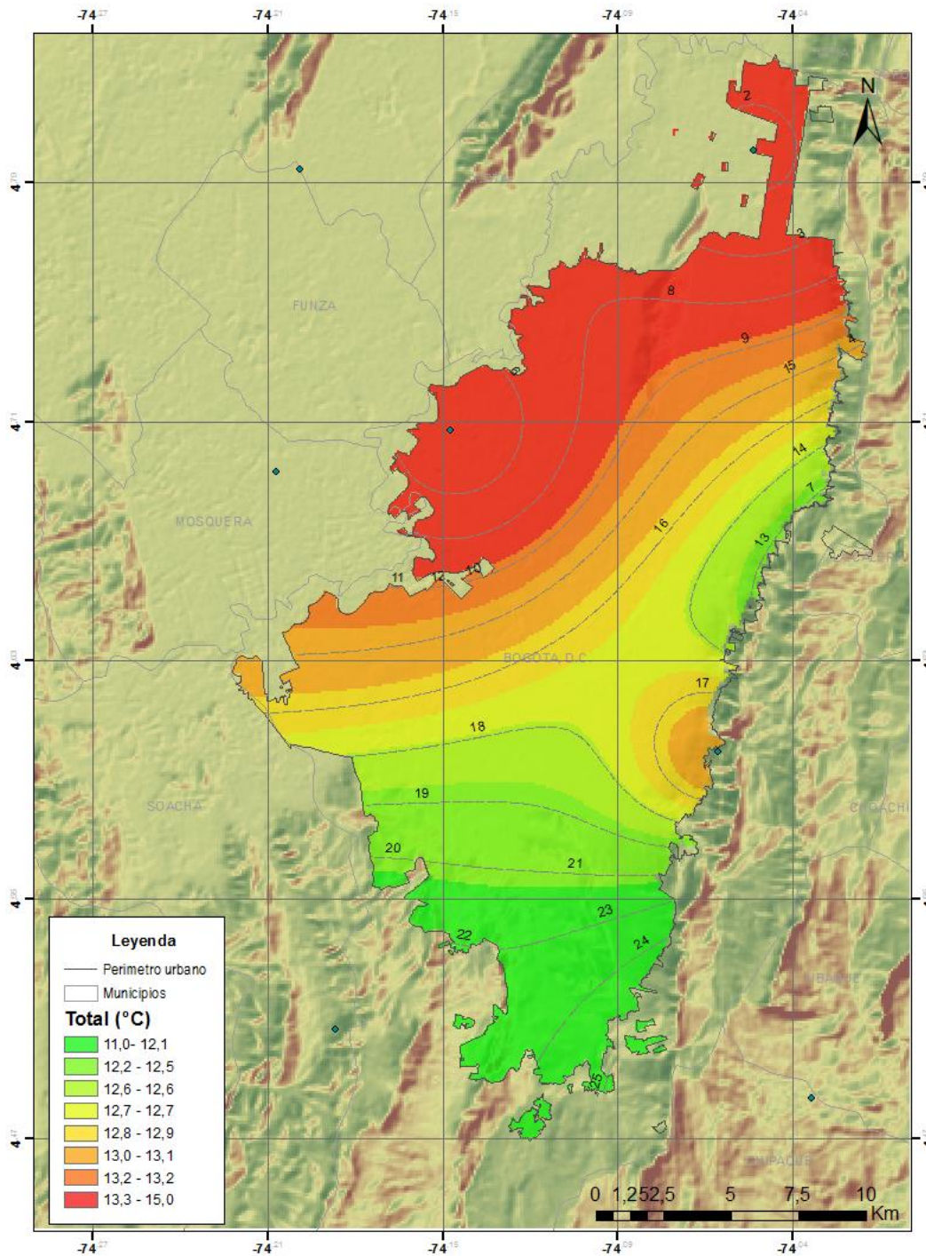
Figura 3-6 Mapa de temperatura media mensual multianual
