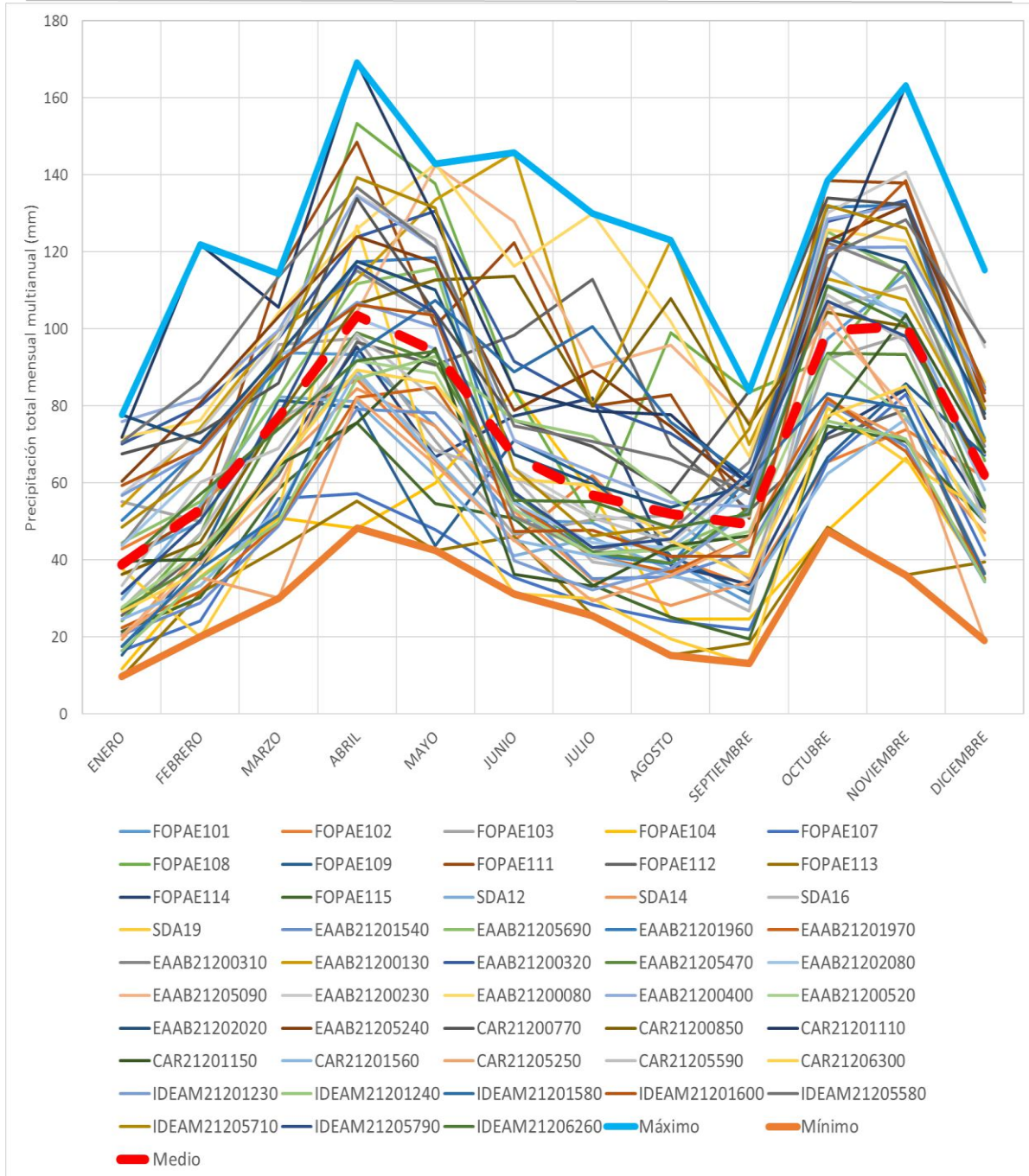
Figura 3-3. Precipitación media, máxima y mínima de las estaciones en el perímetro urbano del distrito
