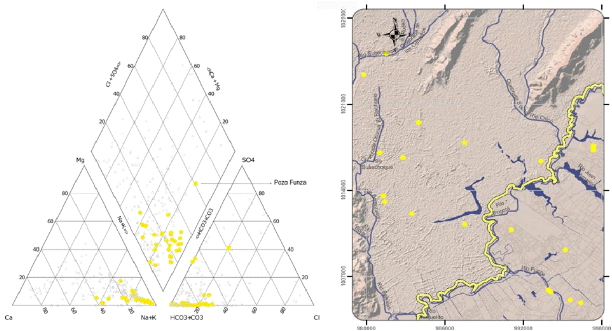
Figura 3-24 Tipos de agua encontrados en los puntos de agua que atraviesan la formación Subachoque
