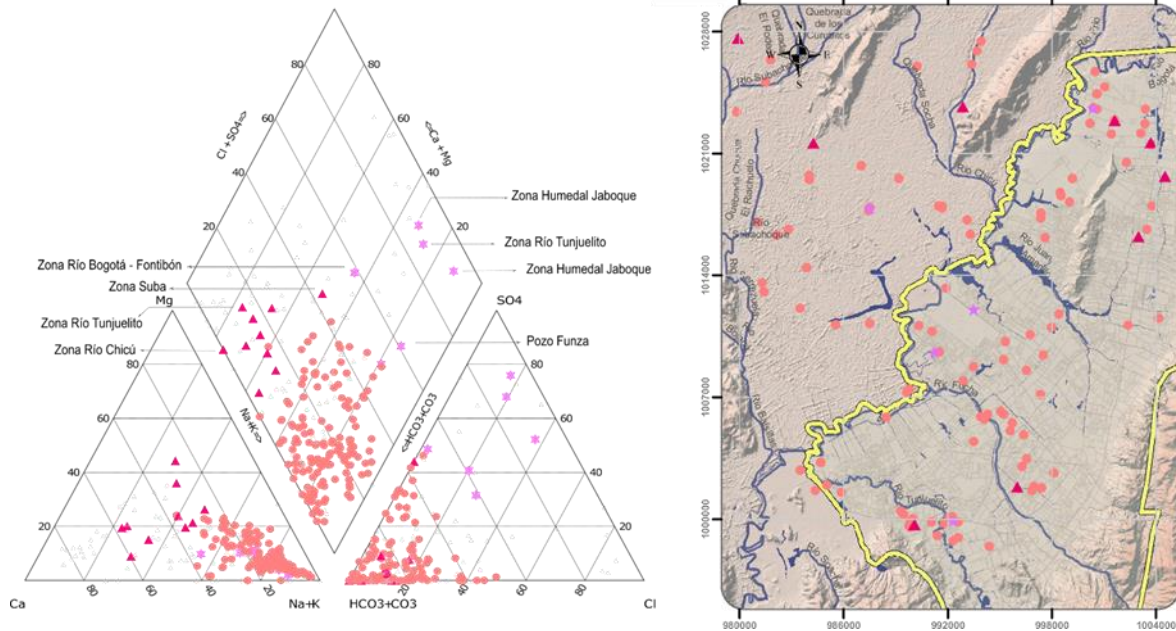
Figura 3-23 Tipos de agua encontrados en los puntos de agua que atraviesan la formación Sabana
