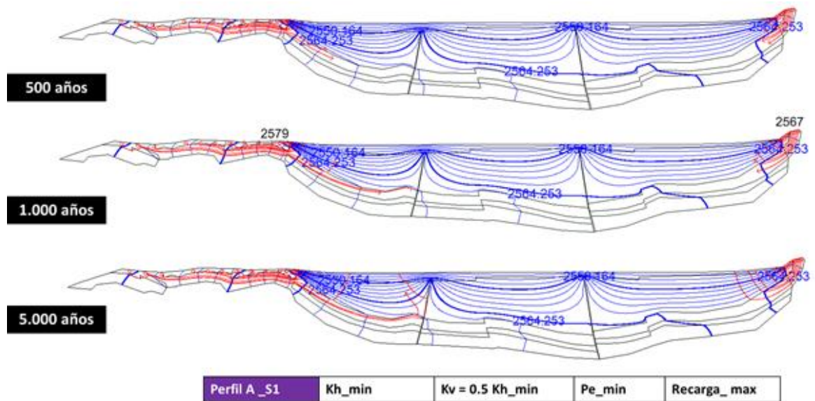
Figura 4-43. Conectividad Regional del acuífero de Bogotá
