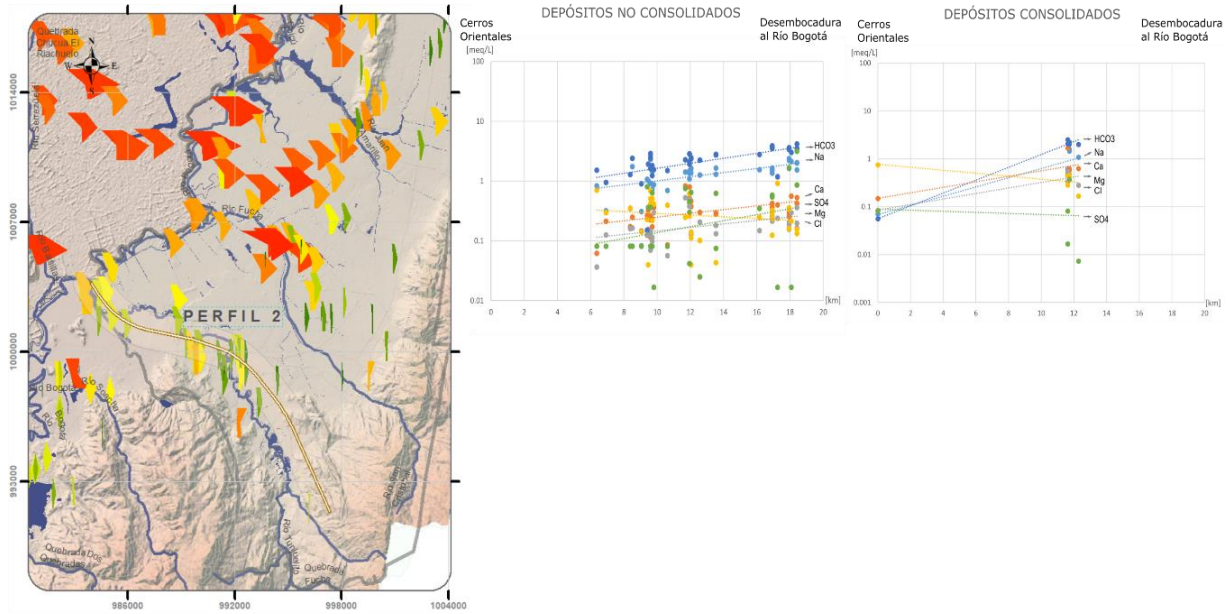
Figura 3-27 Perfil hidrogeoquímico No. 2
