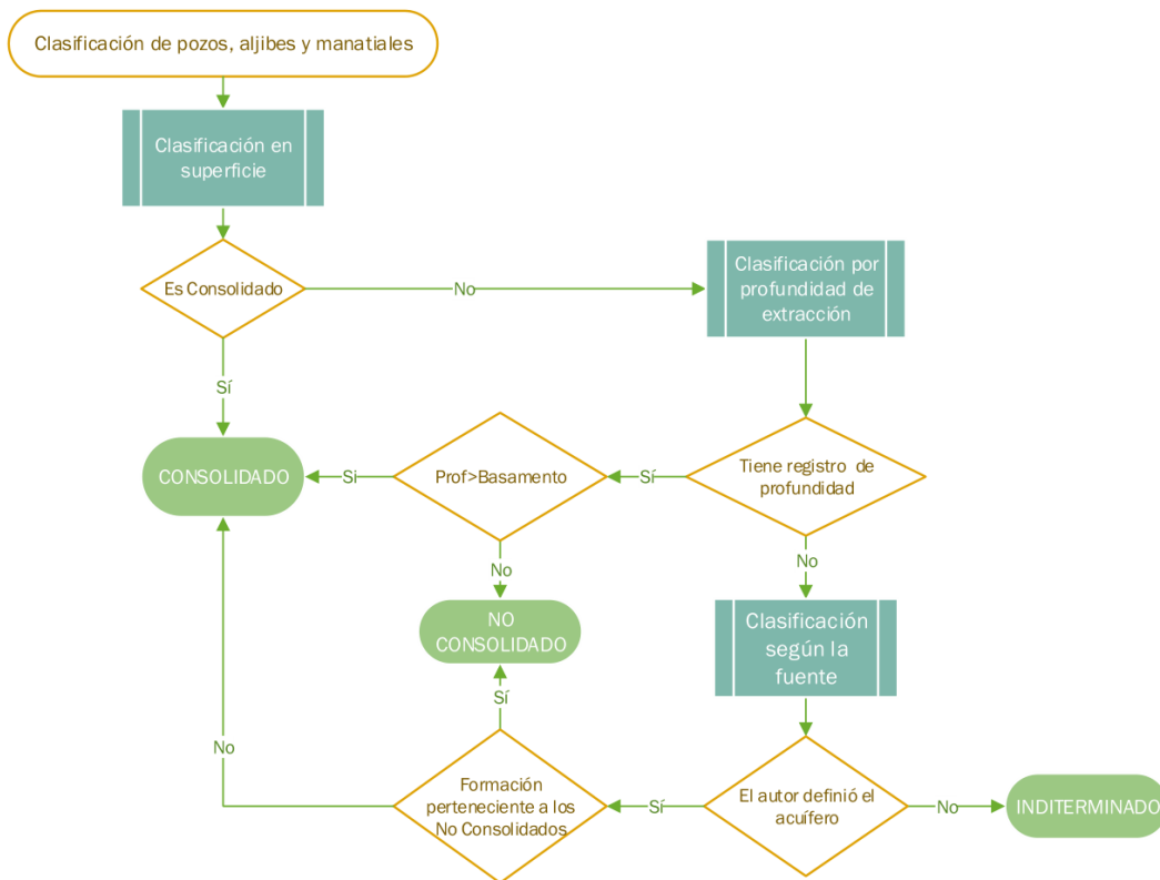
Figura 4-3 Clasificación de pozos, aljibes y manantiales en los depósitos consolidado y no consolidado
