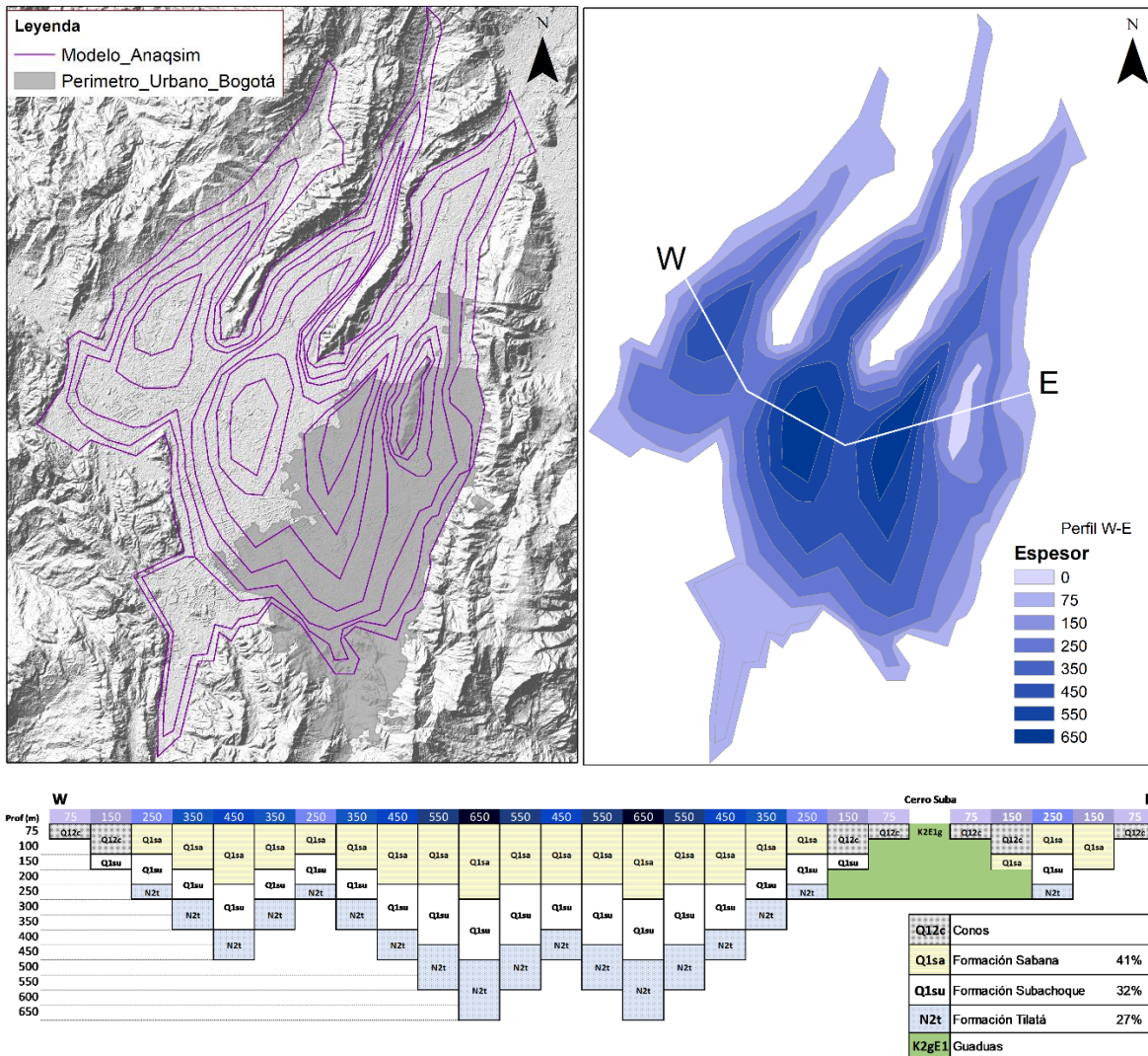
Figura 17 Esquema de la geometría del modelo analítico 3D
