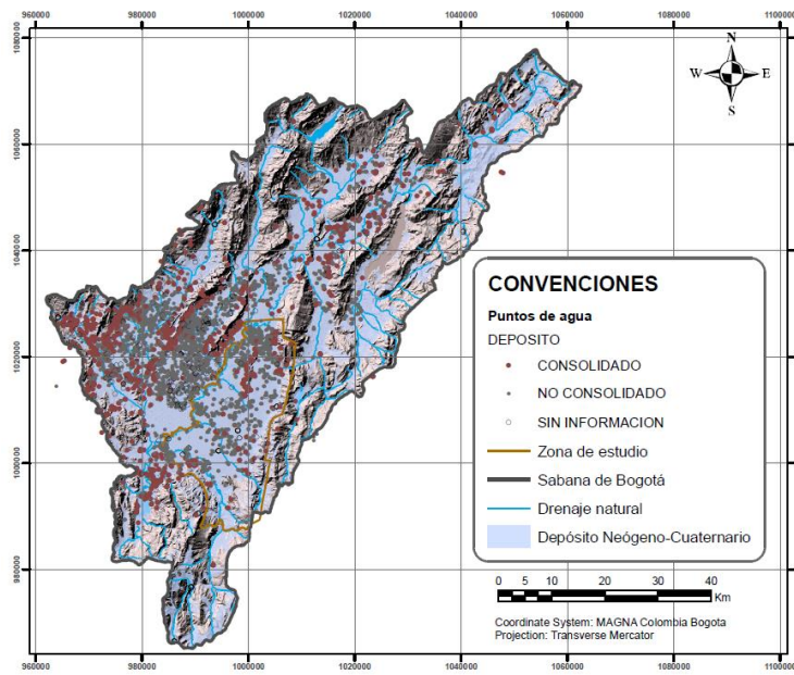
Figura 4-5. Base de datos de puntos de agua clasificados según el depósito de extracción
