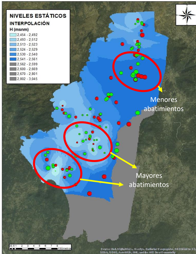
Figura 5-3 Niveles (msnm) interpolados con los datos de los reportes (SDA 2013 y, UNAL 2003) usando un kriging simple con la herramienta geoespacial de ArcGis.
