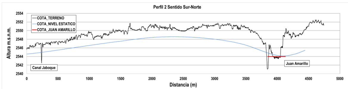
Figura 5-15 Perfil 2 sentido Sur-Norte. Canal Jaboque y Humedal Juan Amarillo A) DEM inicial B) DEM corregido.
