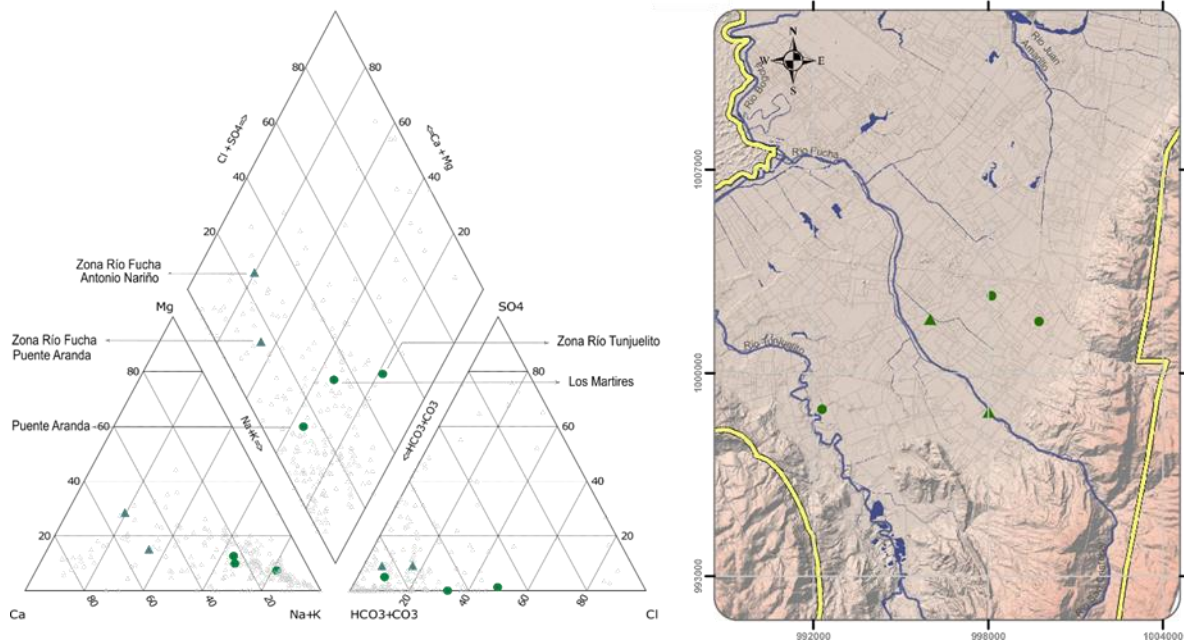
Ilustración 5 Tipos de agua encontrados en los puntos de agua que atraviesan la formación Tunjuelo
