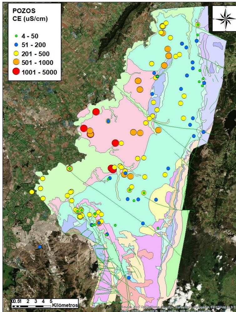
Figura 3-16. Distribución espacial de los valores de Conductividad Eléctrica medida en los pozos
