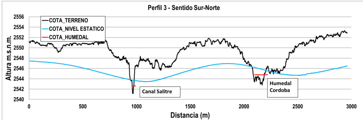
Figura 5-16 Perfil 3 sentido Sur-Norte. Canal Salitre y Humedal Córdoba.
