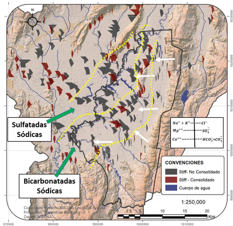
Figura 3-20 Representación gráfica de los diagramas de Stiff para los depósitos consolidados y no consolidados localizados en la zona de estudio
