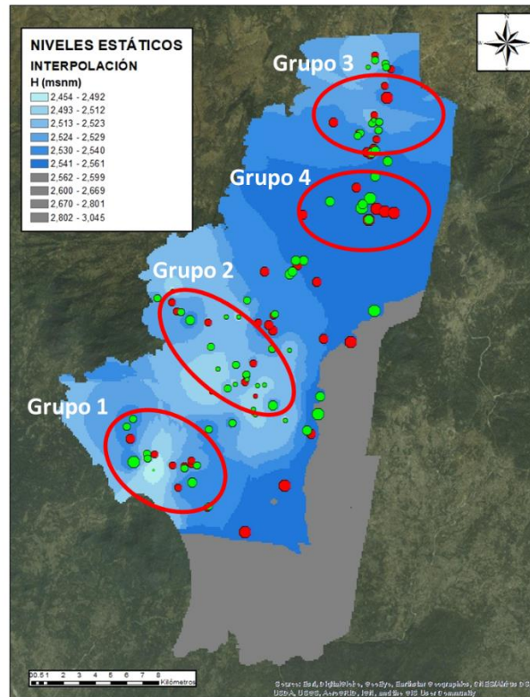
Figura 5-4 Sectorización de los niveles en función de los abatimientos. Esto se hace para realizar el análisis de la evolución temporal del nivel.
