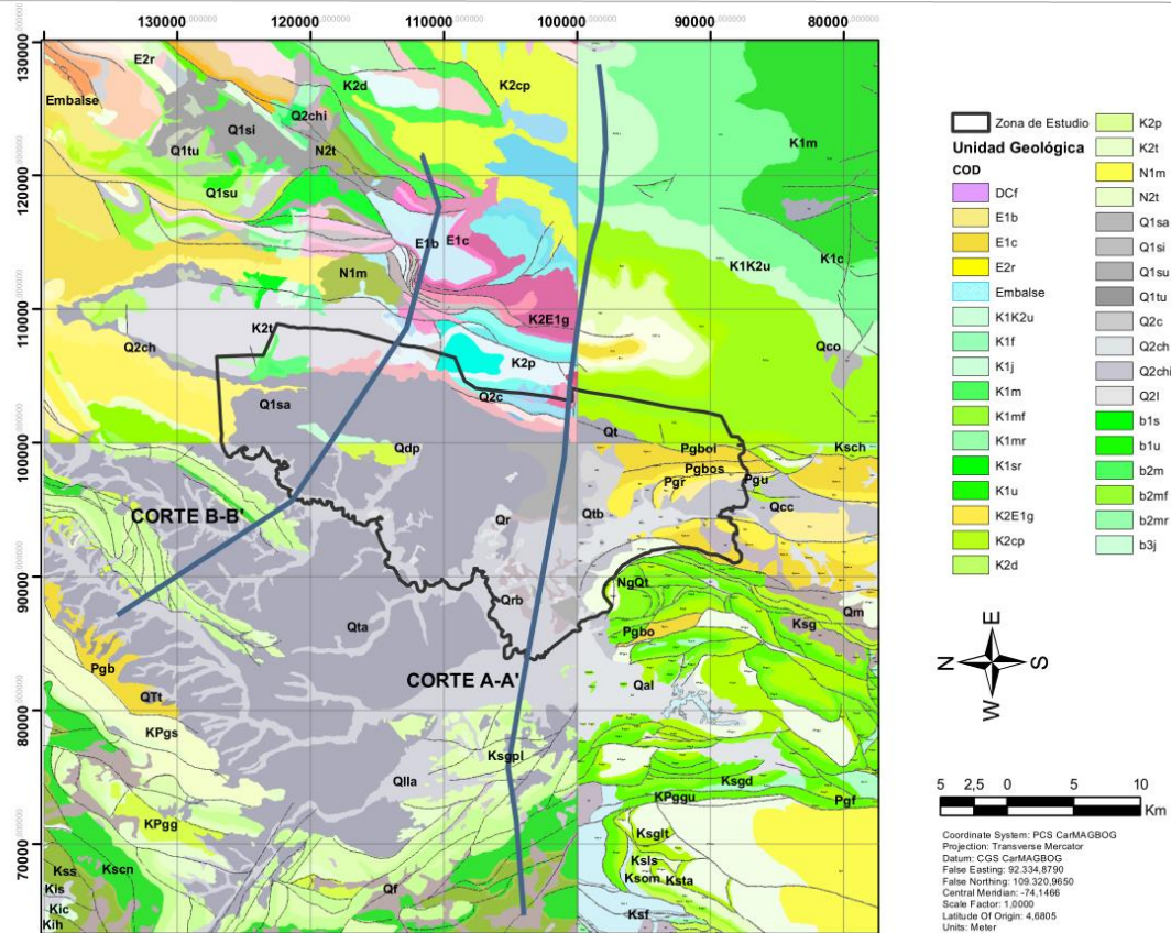
Figura 4-8. Representación de los perfiles en planta sobre los mapas geológicos (227, 228, 246 y 247)
