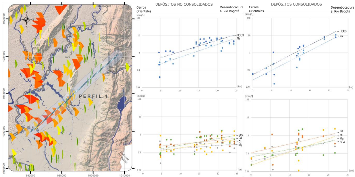
Figura 3-26 Perfil hidrogeoquímico No. 1
