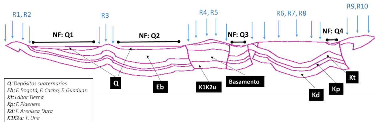
Figura 4-12. Dominio y representación del modelo analítico de flujo 2D, perfil geológico B-B'
