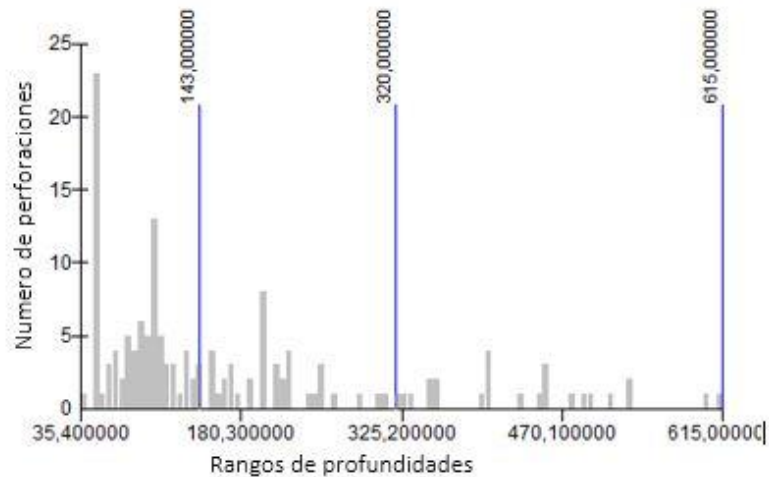
Figura 4-24. Detalle de los rangos de profundidad con más información respecto al número de perforaciones
