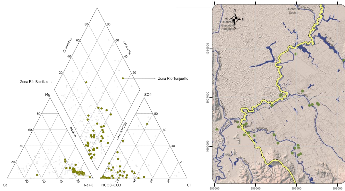
Figura 3-22 Tipos de agua encontrados en los puntos de agua que atraviesan la formación Chía
