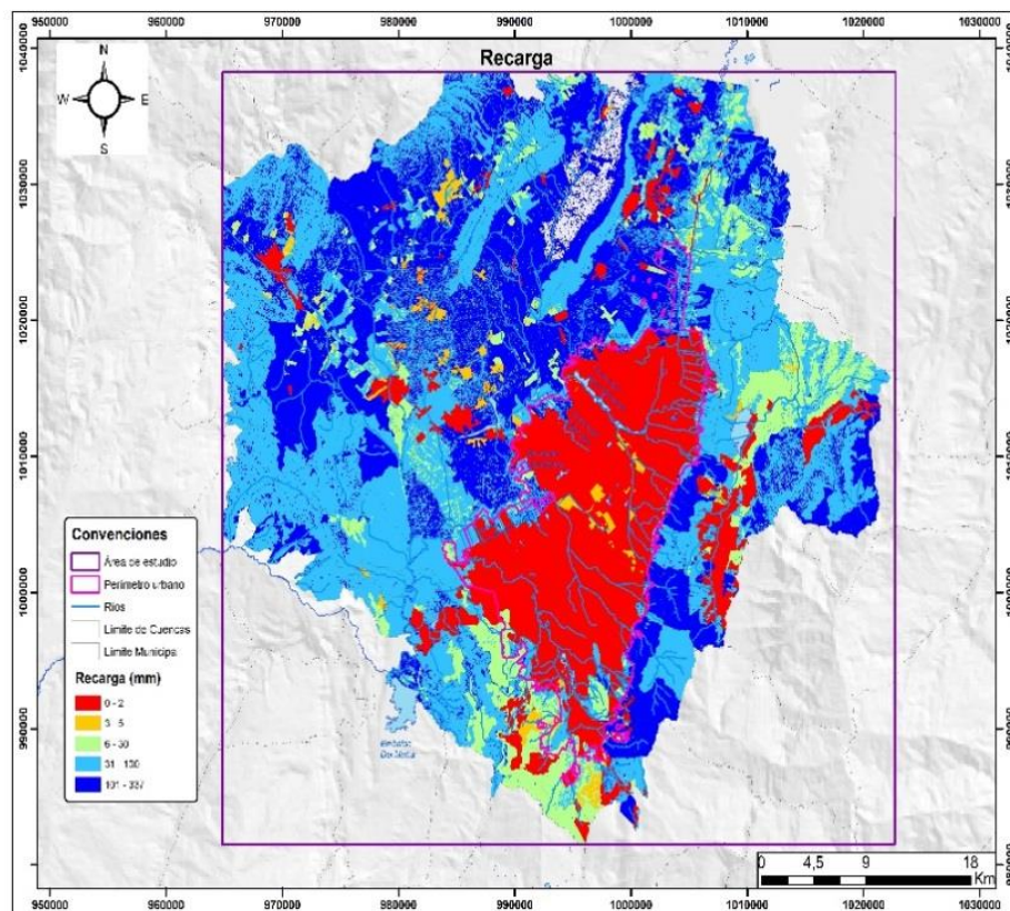
Figura 4-37 Recarga natural (mm/año)
