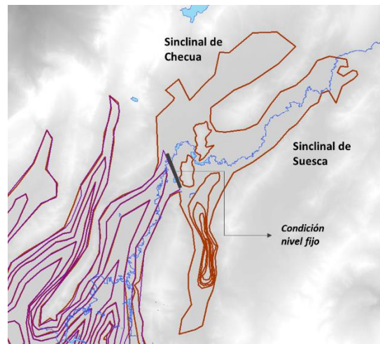
Figura 20 Condición de frontera nivel fijo
