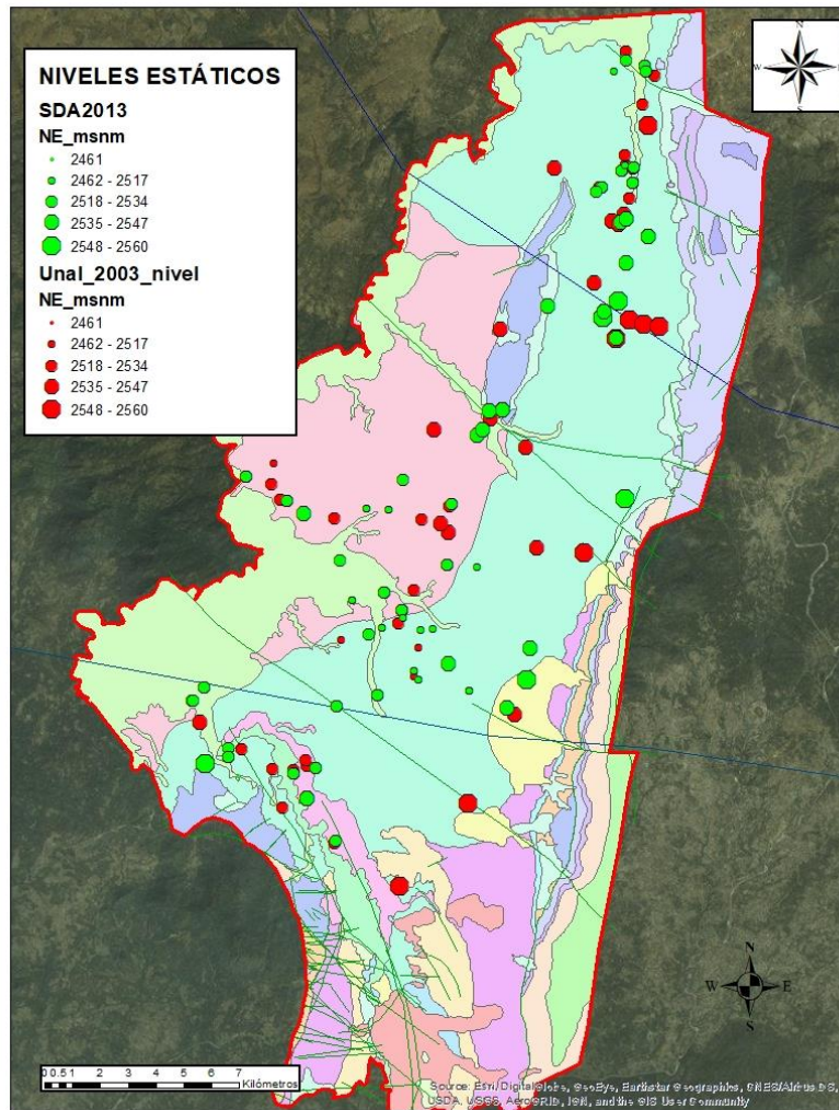
Figura 5-2 Comparación de los niveles estáticos puntuales de los reportes (SDA 2013 y, UNAL 2003).
