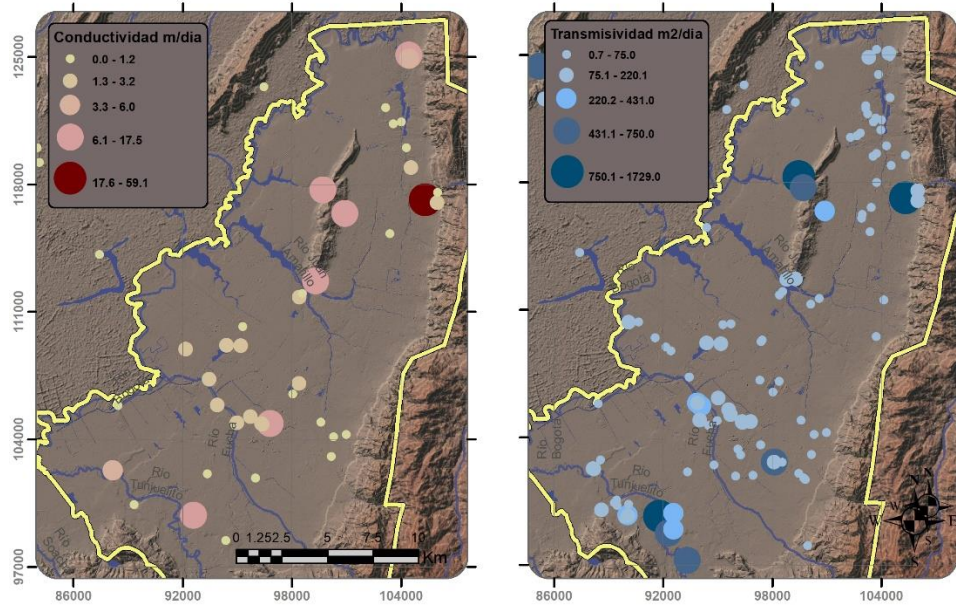
Figura 4-5. Puntos de agua con información de conductividad ( K ) y transmisividad ( T )
