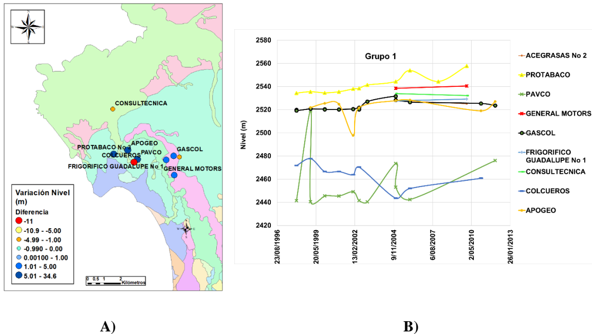
Figura 5-5. Localización y evolución temporal de los pozos localizados en el grupo 1. A). Localización y el valor puntual entre la diferencia de nivel medido entre la más reciente a la más antigua, B). Evolución temporal de los niveles.
