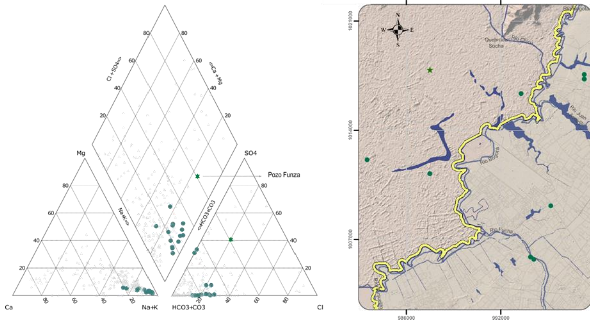
Ilustración 6 Tipos de agua encontrados en los puntos de agua que atraviesan la formación Tiltatá
