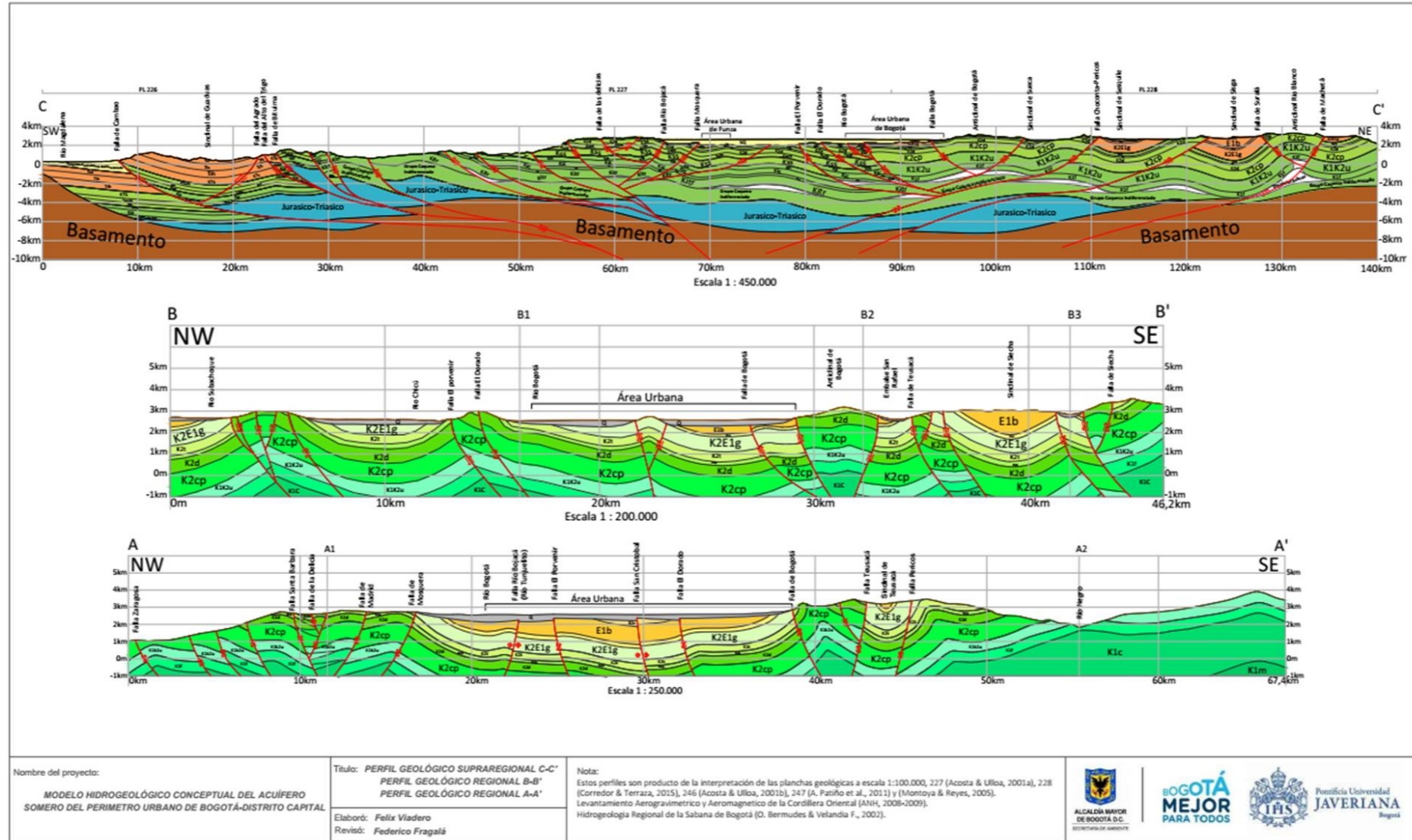
Figura 3-12. Perfiles regionales AA', BB' y supraregional CC'
