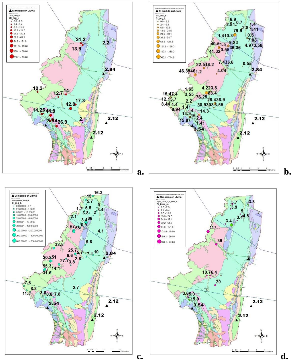
Figura 3-18. Medidas de Cl- en las campañas de a) Jica 2009; b) Jica 2003; c) Hidrogeocol 2000 y d) Ingeominas 1998-2000
