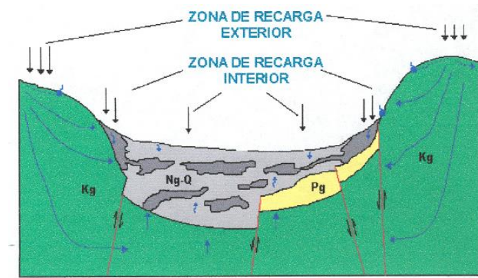
Figura 1-3. Modelo hidrogeológico esquemático de la cuenca de la sabana de Bogotá.
