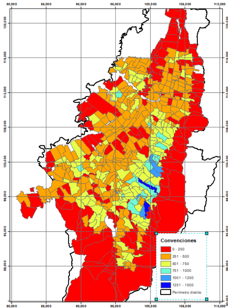
Figura 4-41: Recarga artificial en mm/año
