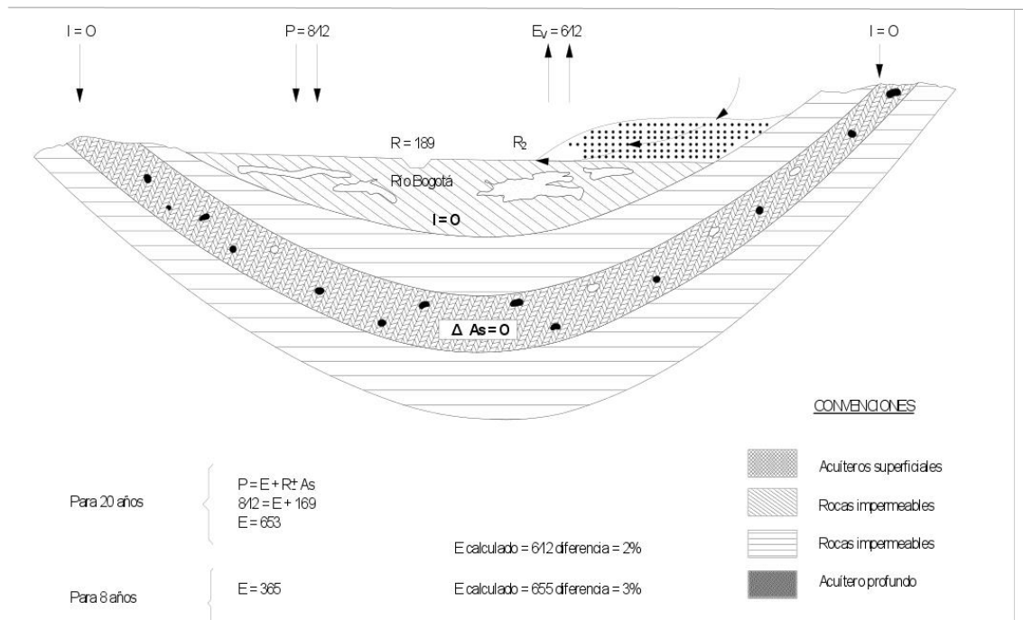
Figura 1-1 Esquema conceptual del balance hídrico
