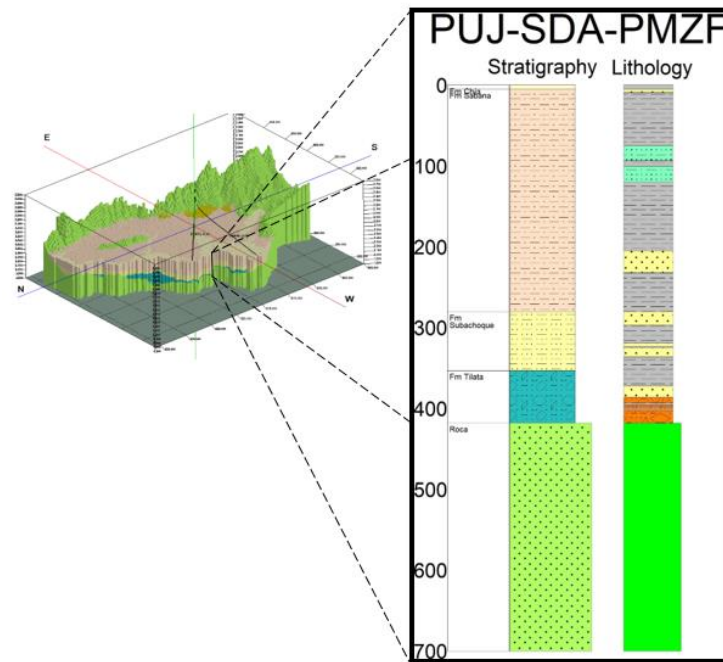
Figura 4-34. Columna litológica y estratigráfica pozo PUJ-SDA-PMZF
