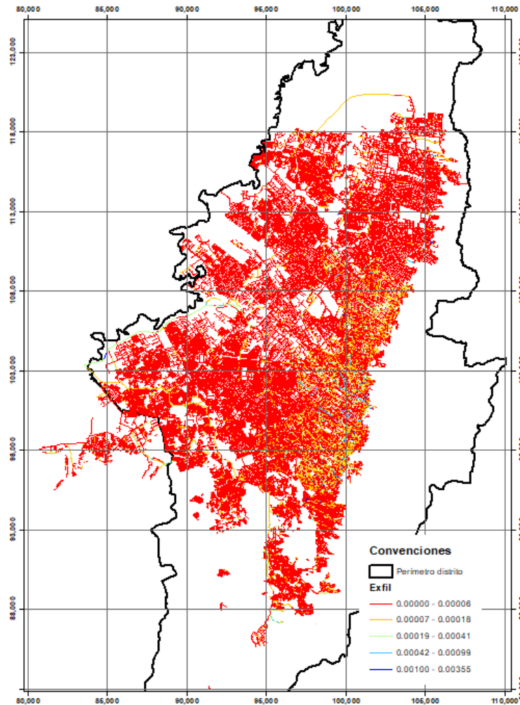
Figura 4-39: Exfiltraciones en m 3 /s de la red de alcantarillado sanitario
