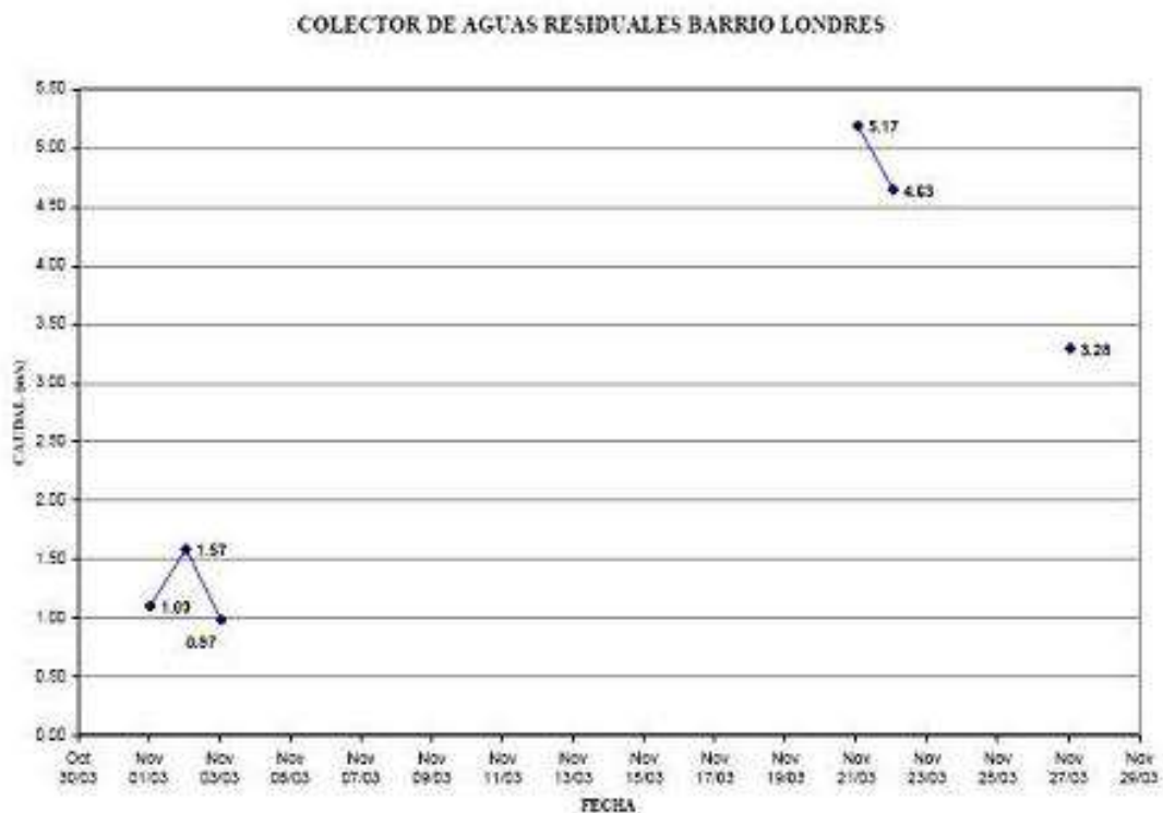
Figura 13. Caudal reportado para el Colector de aguas residuales, Barrio Londres (Geodesia por Satélite & FHLC, 2004).
