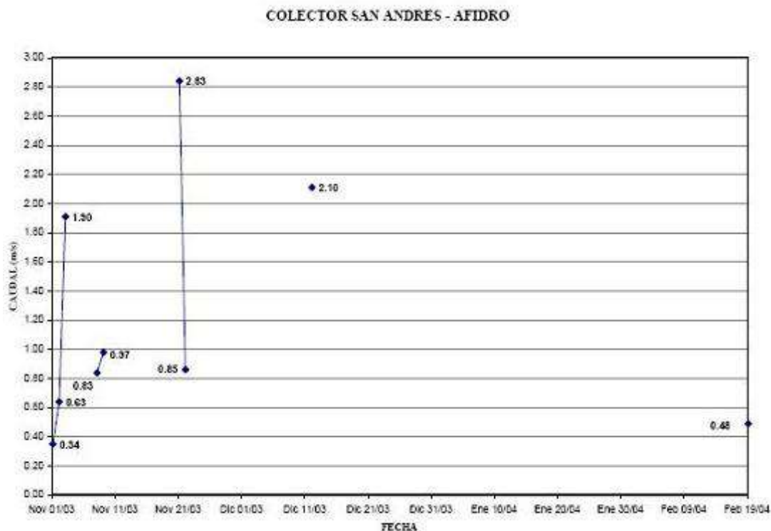
Figura 16. Caudal reportado para el Colector de aguas residuales, San Andrés - Afidro (Geodesia por Satélite & FHLC, 2004).
