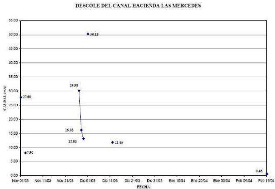
Figura 15. Caudal reportado para el Colector de aguas residuales, Canal Hacienda Las Mercedes (Geodesia por Satélite & FHLC, 2004).
